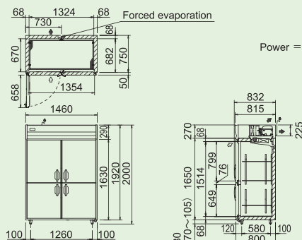
SRR-1581HP(E)
