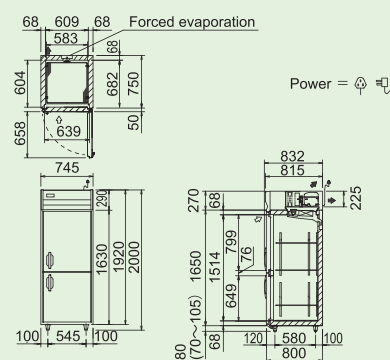
SRR-781HP(E)
