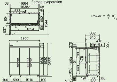
SRR-1881HP(E)
