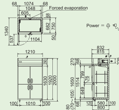
SRR-1281HP(E)
